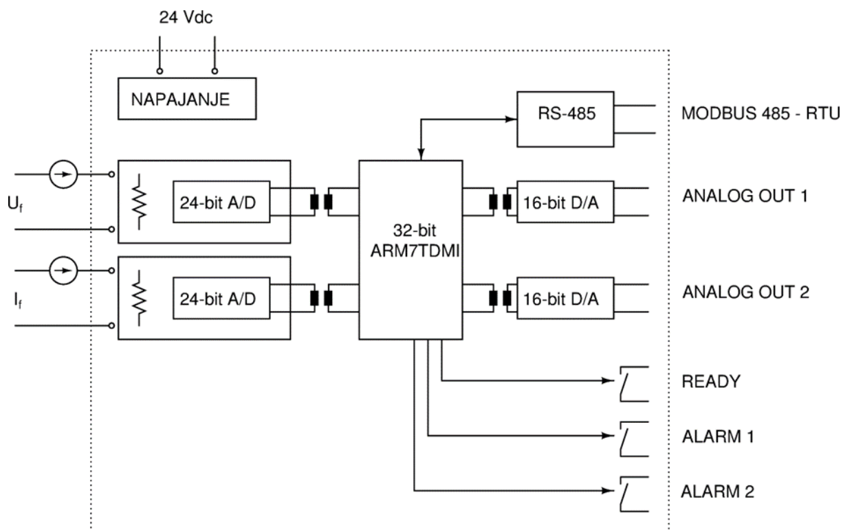
Слика 1: Блок-шема модула
