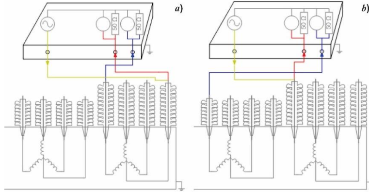
SL.3 – Principijelna šema izvođenja mjerenja frekventnih odziva na dvonamotajnom transformatoru
