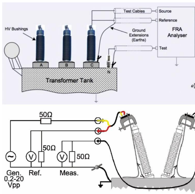
Sl. 2 - Način spajanja mjernih kablova između uređaja M5400 i priključaka transformatora
