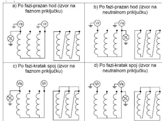
SL. 4 – Načini priključena pobudnog sinusnog napona na krajeve namota
