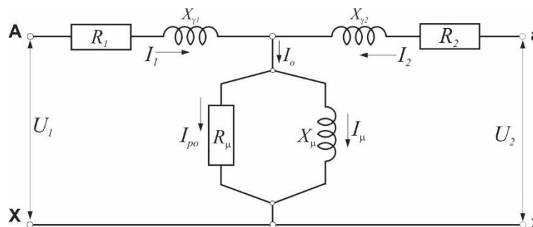
SL. 5 – Ekvivalentna T šema transformatora
